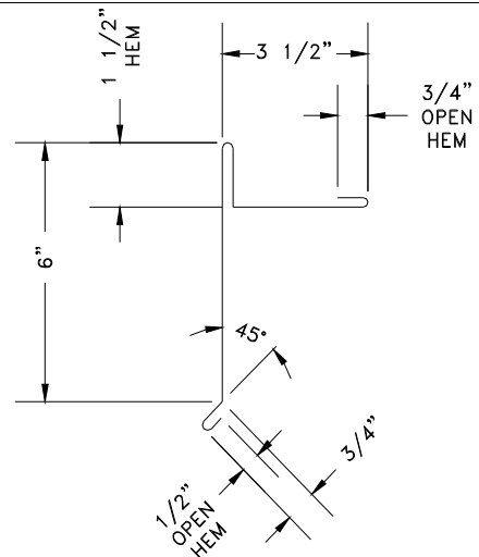
RAKE
